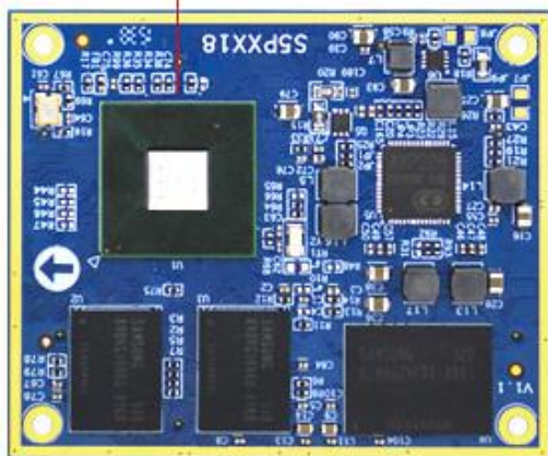
S5P四核4418与八核6818底板兼容
