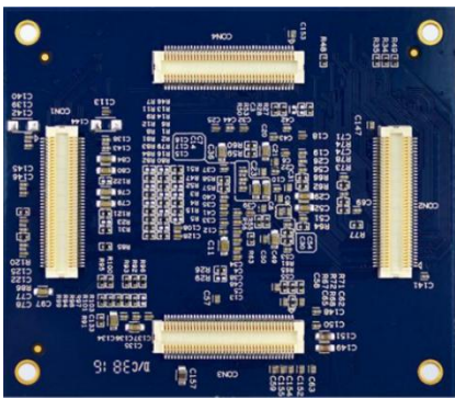
核心板背面
